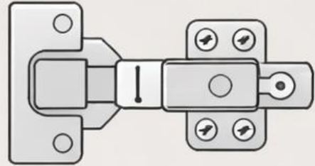
8° Crank Hinge
