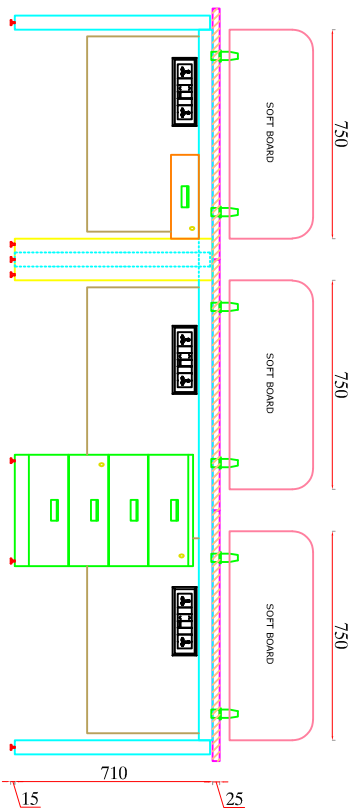
ELEVATION
