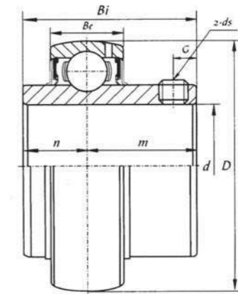
UC 200 (normal-duty)
