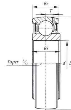
UK 200 (normal-duty)
