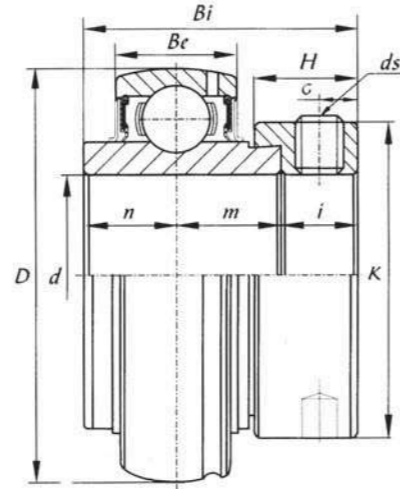
HC 200 (normal-duty)
