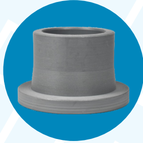
Long Neck Stub End Mfg Range : 20 mm OD to 500 mm OD
