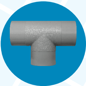
Tee ( Spigot Type ) ( 6 Kg. & 10 Kg. ) Mfg Range : 63 mm OD to 315 mm OD
