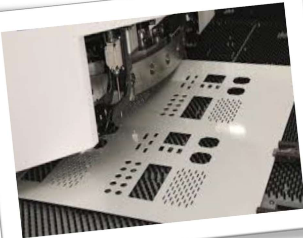
TURRET PUNCH PRESS
